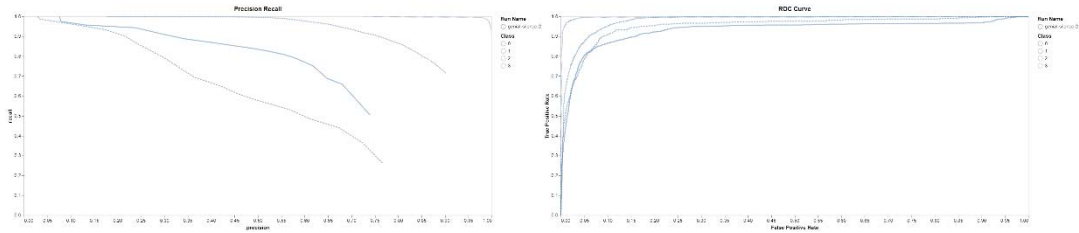
圖十二：XLNet 模型最佳效能評估分析 (Precision Recall & ROC curve)
