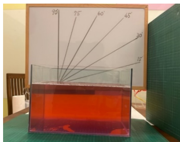
圖 3-1：在調配好泡泡水的水族箱側邊固定標記好角度的板子
