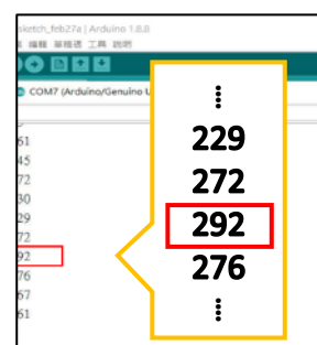
圖 5-2-3-3：序列埠監控視窗圖，最大受力值為 292 gw
