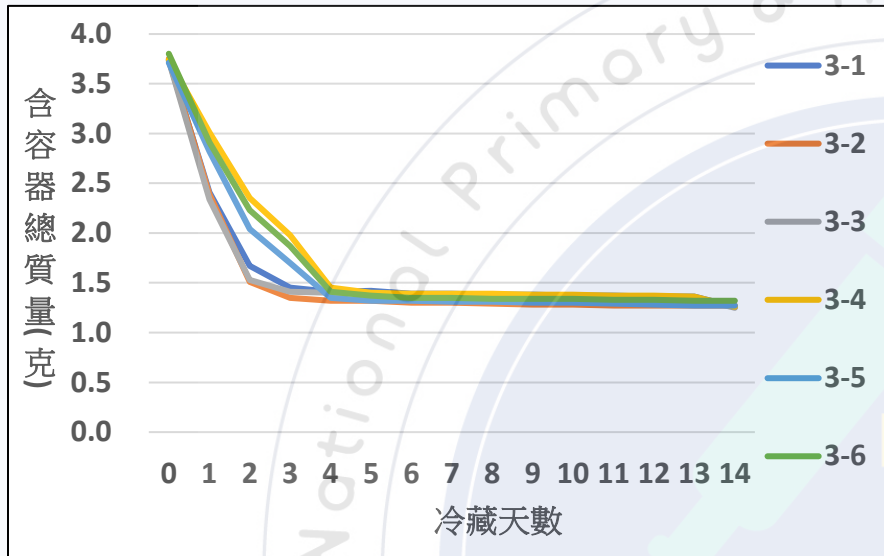
圖6 以鋁箔小碟當容器薄膜質量與冷藏時間的關係圖
