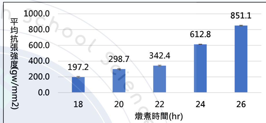
圖10 燉煮時間對製得的魚鱗薄膜抗張強度的關係圖
