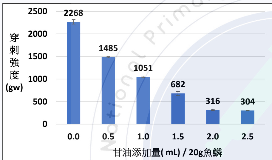
圖13 不同甘油量，對魚鱗薄膜穿刺強度的關係圖
