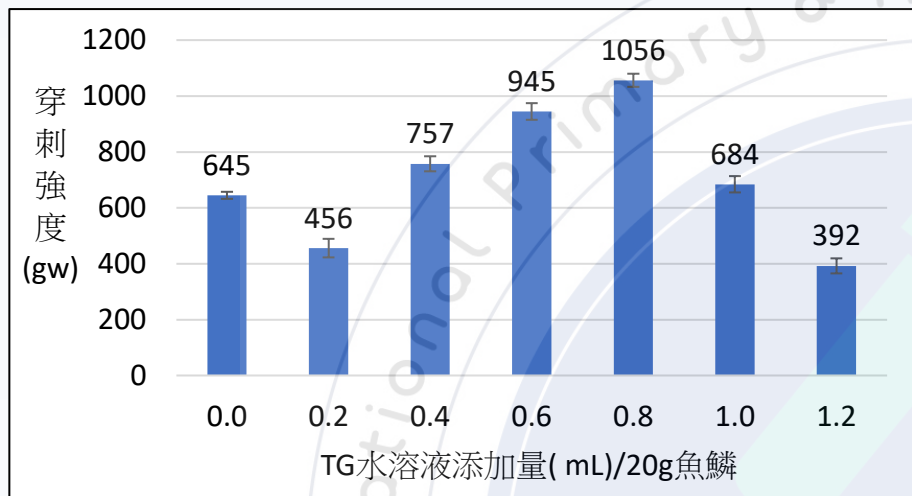
圖16 不同量的TG水溶液量對魚鱗薄膜穿刺強度的影響
