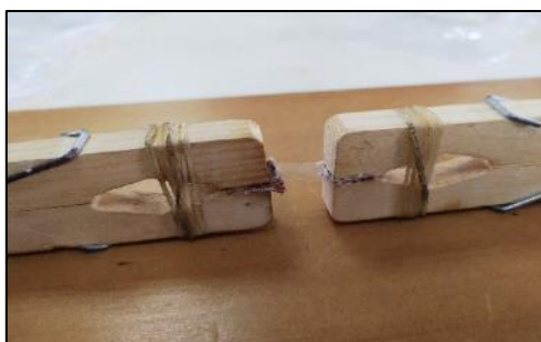
圖 5-2-2-2 抗張強度測量實際圖
