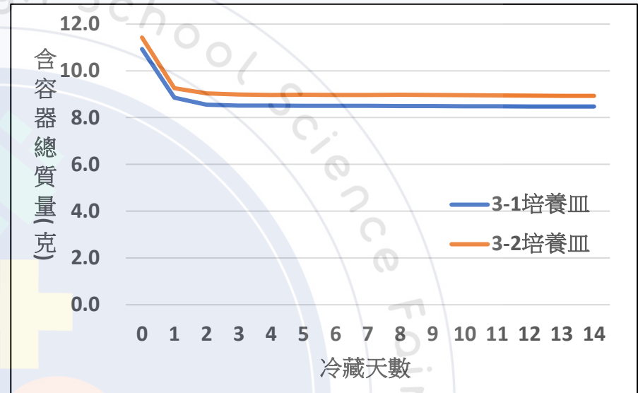
圖7 以培養皿當容器薄膜質量與冷藏時間的關係圖
