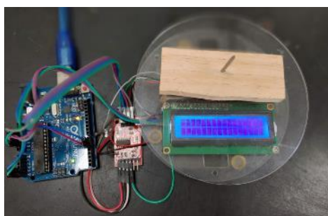
圖 5-2-3-2：Arduino 的 HX711 電子天平實物圖
