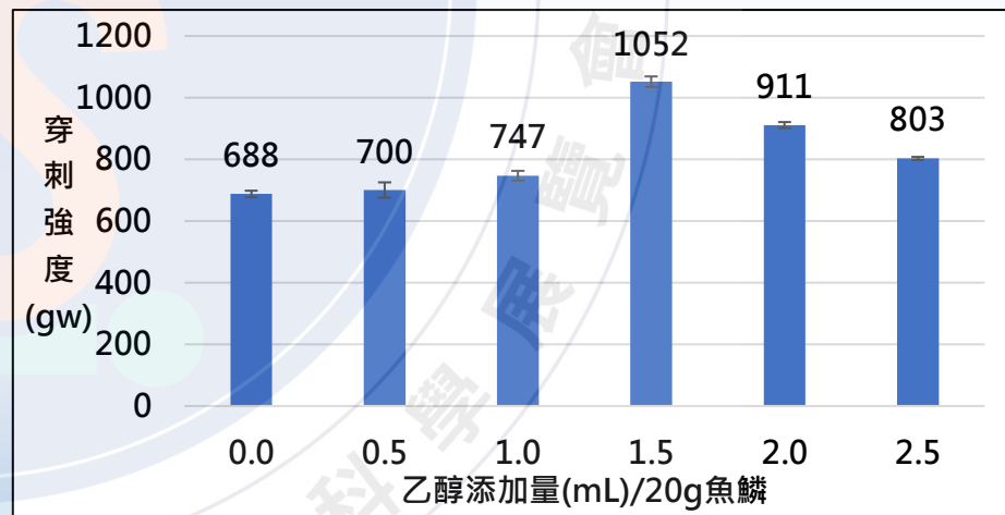
圖12 不同乙醇的量，對魚鱗薄膜穿刺強度關係圖
