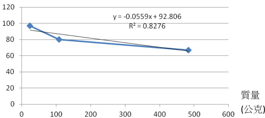
圖 6-4 質量與最小成膜高度之關係
