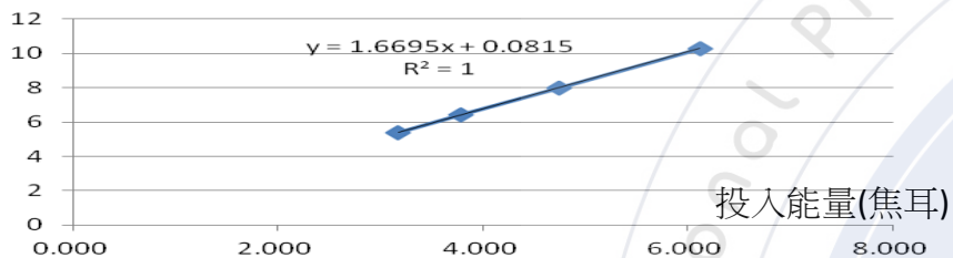
圖6-9 484公克龜甲石釋放能量與形成水膜高度關係
