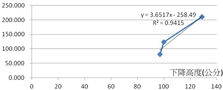
圖 6-15 24 公克中彈珠下降高度與空氣甜筒體積關係
