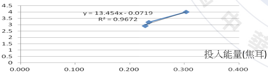
圖6-11 24公克中彈珠釋放能量與形成水膜高度關係
