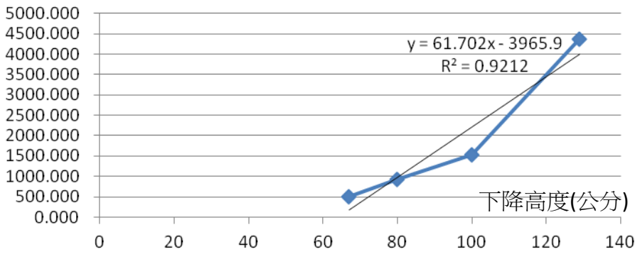
圖 6-13 484 公克龜甲石下降高度與空氣甜筒體積關係
