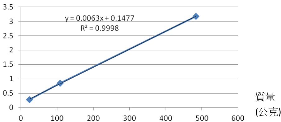
圖 6-5 質量與最小成膜能量(焦耳)之關係
