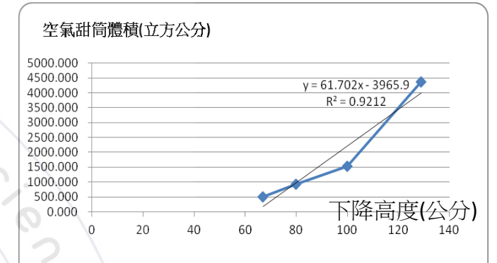
圖6-15 484公克龜甲石下降高度與空氣甜筒體積關係
