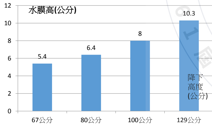
圖6-1 龜甲石之降下高度與水膜高度圖
