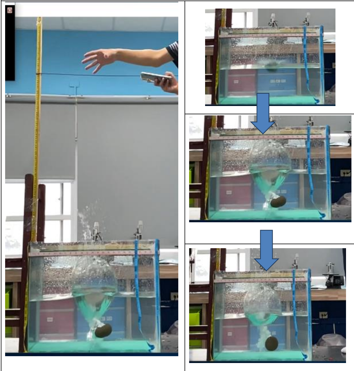
實驗方式圖解
