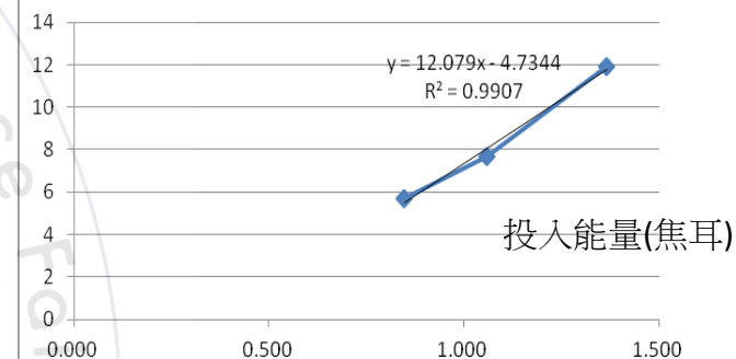
圖6-13 108公克大彈珠釋放能量與最深水深關係
