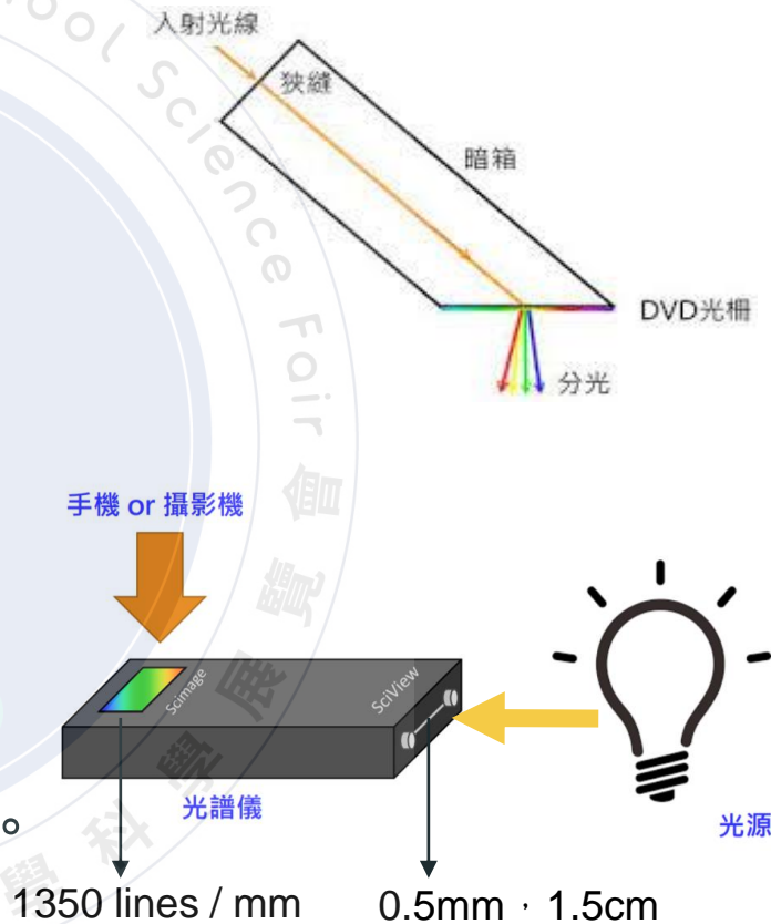
圖2 手機光譜儀示意圖[7]
