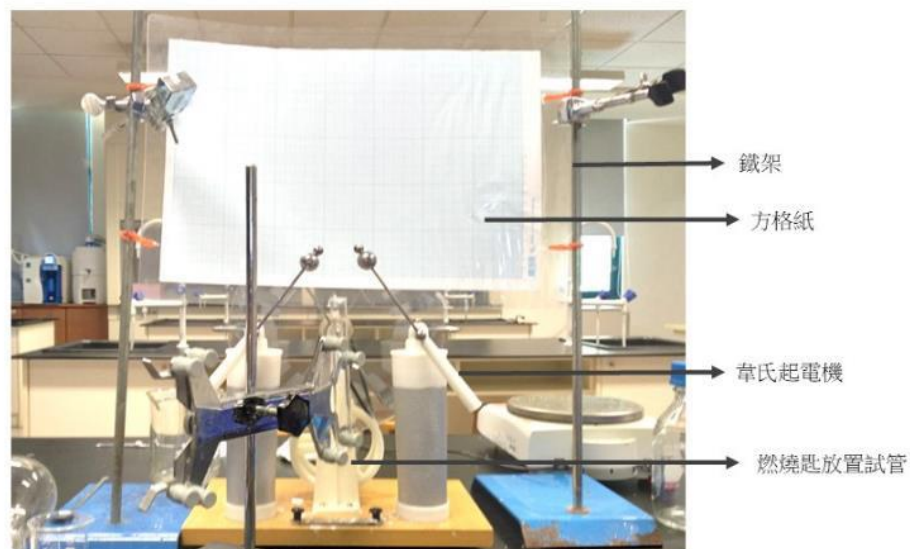
圖 8 焰色偏轉實驗裝置圖
