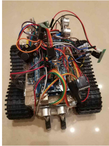
圖 6-1 履帶智能車
