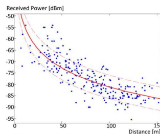
圖 5-15 dBm 與距離的關係圖
