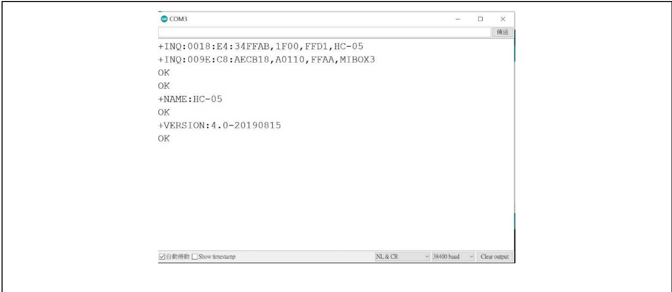
圖 5-16 藍牙信號強度測量過程圖
