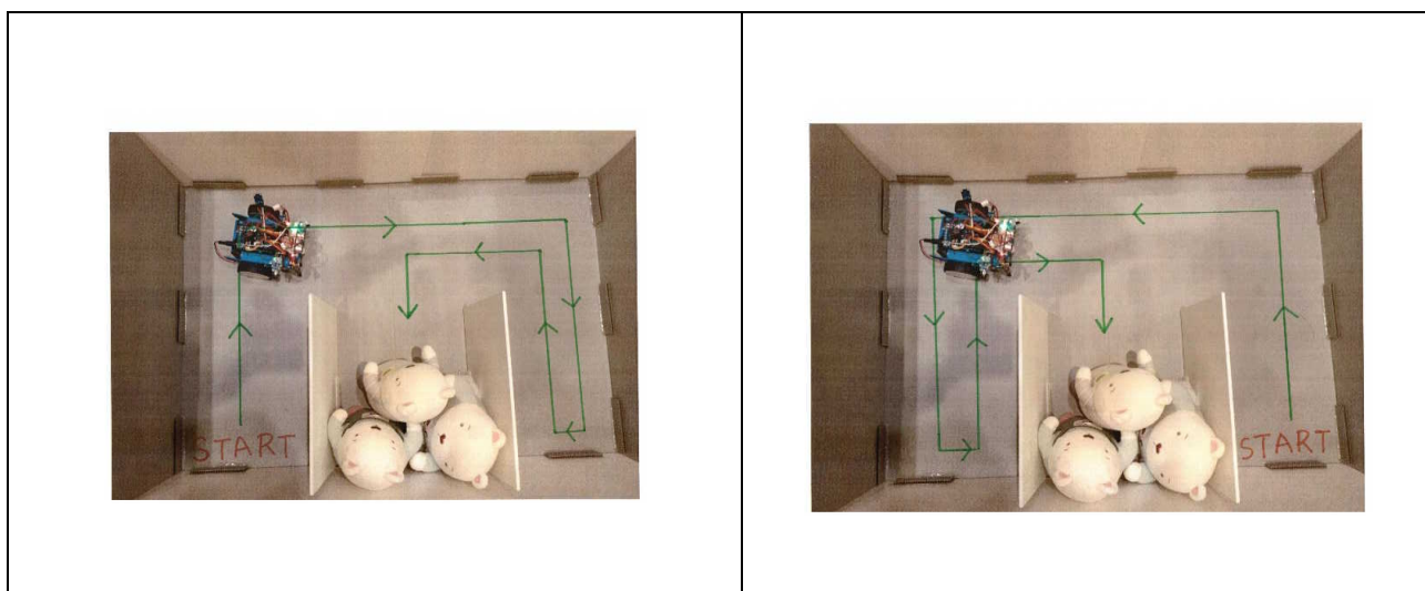
圖 5-10 迷宮(60cm*90cm)右轉法和左轉法測試
